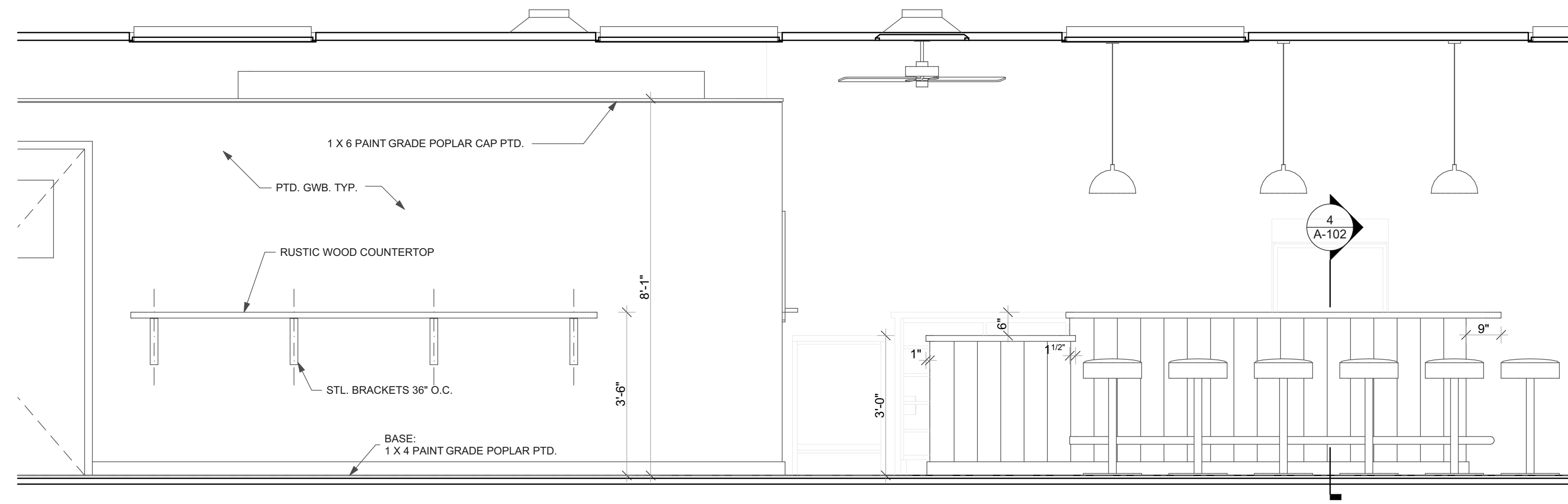
2 A-102 INTERIOR ELEVATION SCALE: 1/2" = 1'-0"
