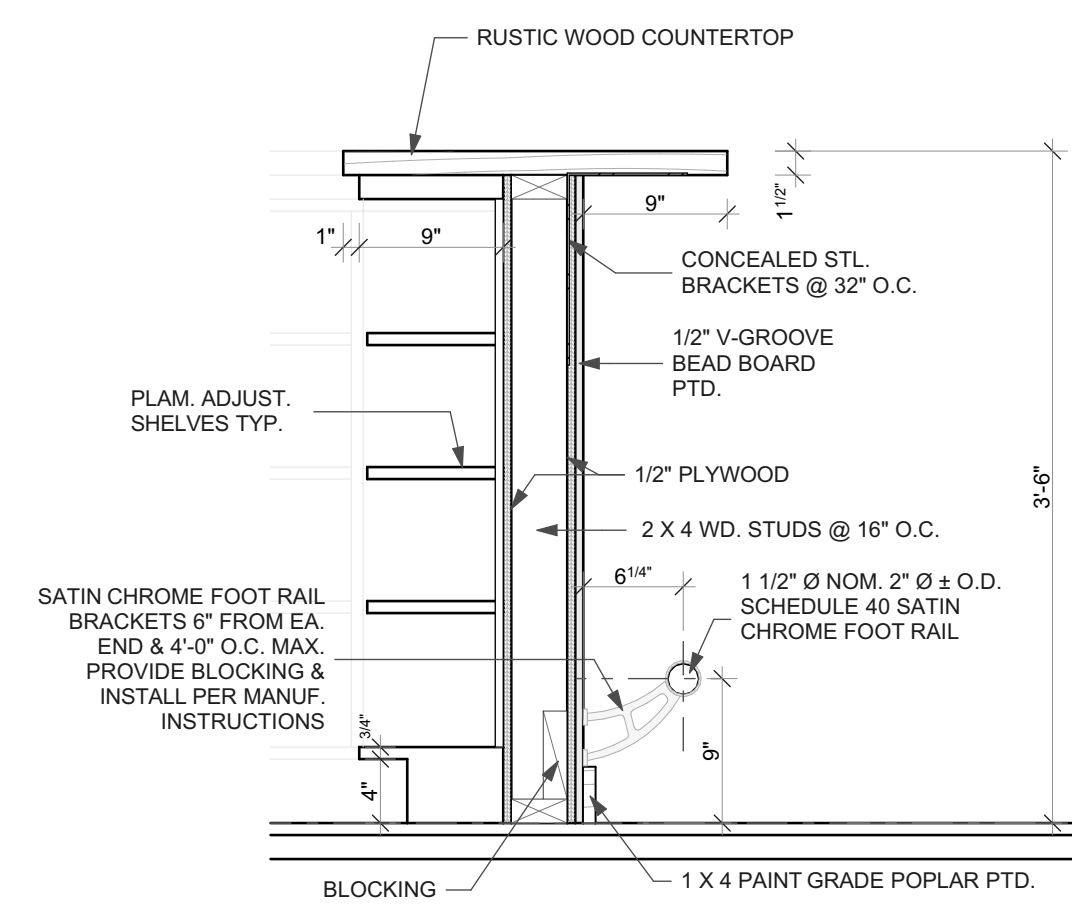
4 A-102 COUNTER SECTION SCALE: 1" = 1'-0"
